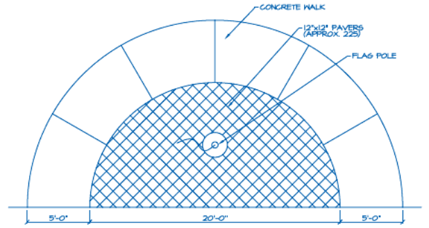
FLAG POLE / PAVER DETAIL SCALE: 1/2"=1'-0"
